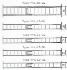
A 型钢质复合铝蜂窝板/A 型复合铝板铝蜂窝板
