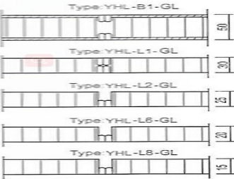
C 型钢质复合铝蜂窝板/C 型复合铝板铝蜂窝板
