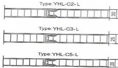
A 型复合铝板铝蜂窝天花板/A 型钢质复合铝蜂窝天花板
